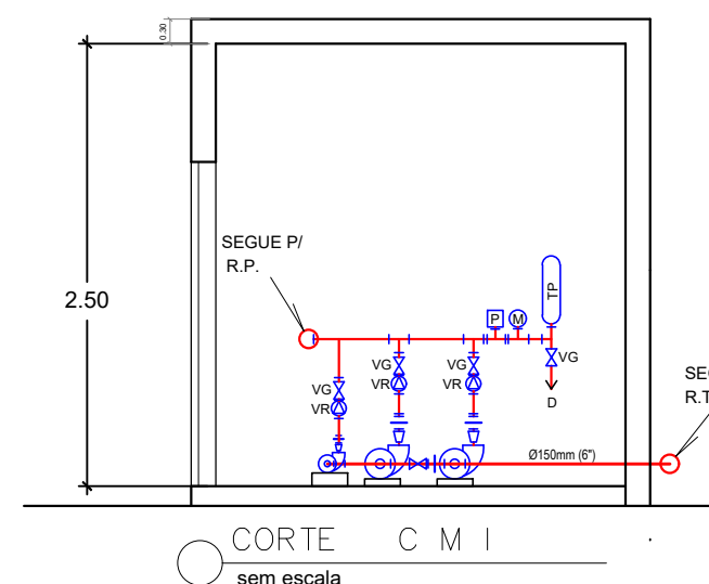
NOTA - SISTEMA DE BOMBAS Bomba Principal: Elétrica Bomba Reserva: Motobomba
