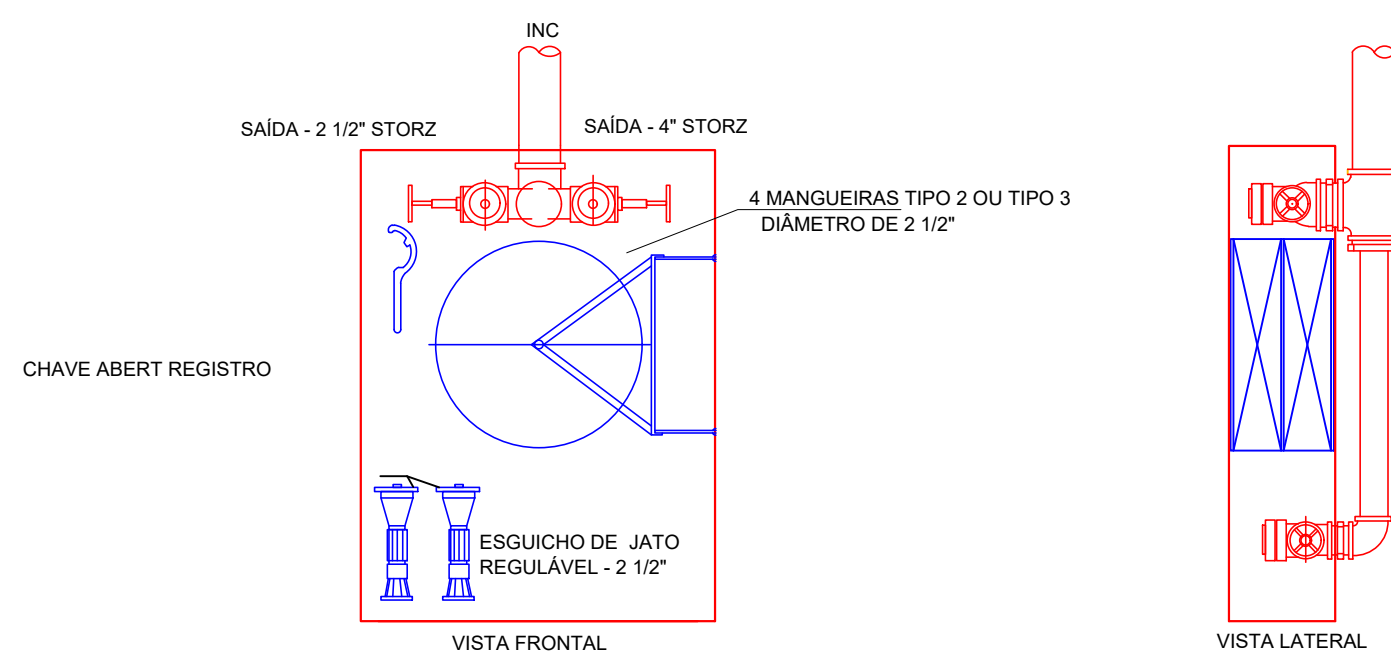
ABRIGO PARA HIDRANTES (HIDRANTE DUPLO) - ALIMENTAÇÃO SUPERIOR
