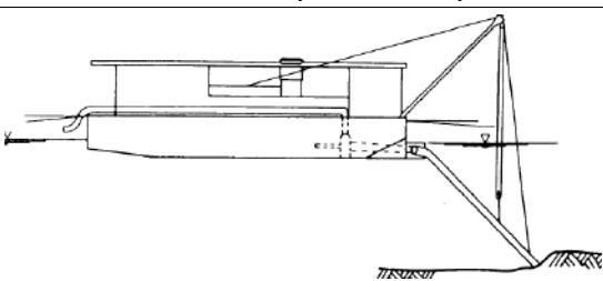
Remoção por Bombeamento de Produto Denso
