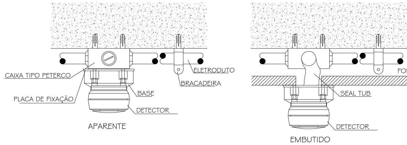
DETALHE DE FIXAÇÃO DE DETECTORES SEM ESCALA
