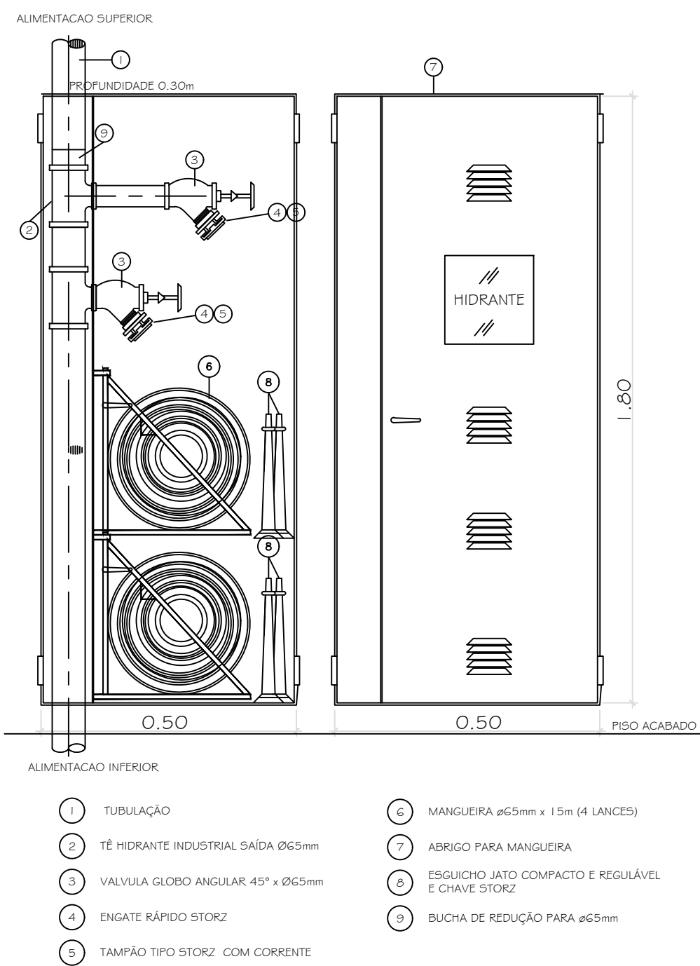
VISTA EXTERNA E INTERNA - HIDRANTE DUPLO SEM ESCALA
