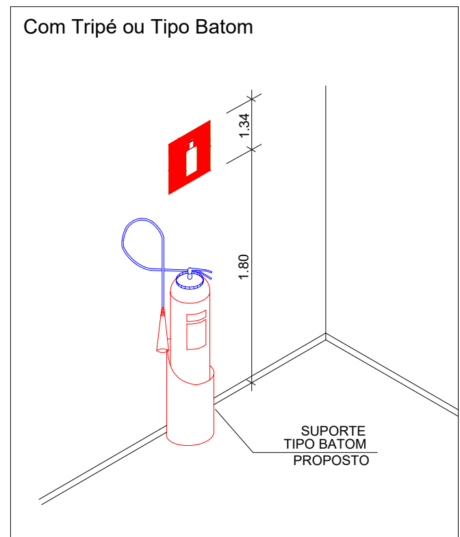
DETALHAMENTO EXTINTORES SEM ESCALA
