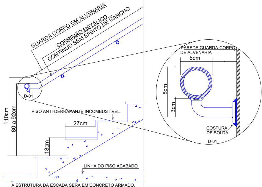
DET. ESCADA / CORRIMÃO / GUARDA CORPO EM ALVENARIA
